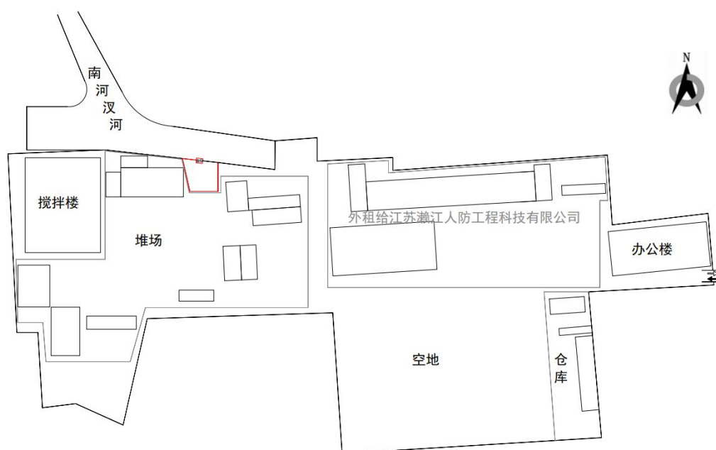
图4-3 厂区平面布置图
